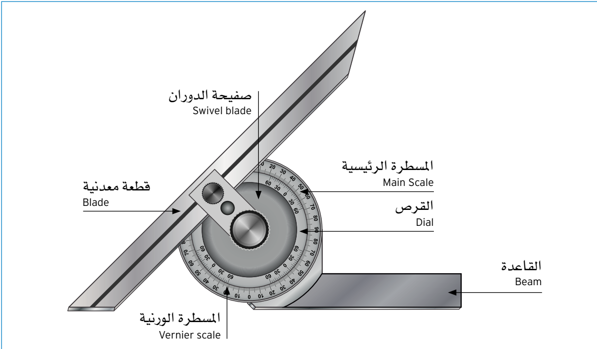
المنقلة المحورية ذات الوردية
