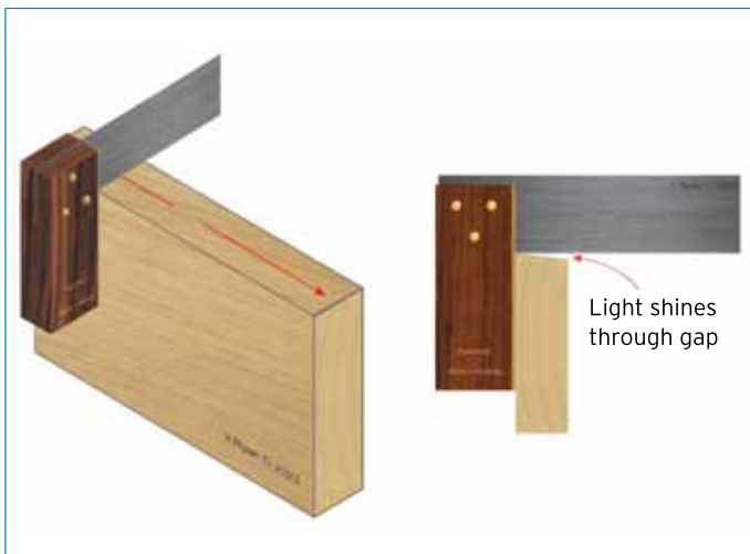
قياس الزاوية القائمة بالمسطرة القائمة
