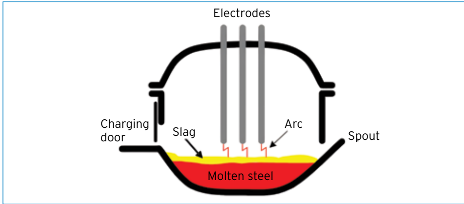
أفران القوس الكهربائي
