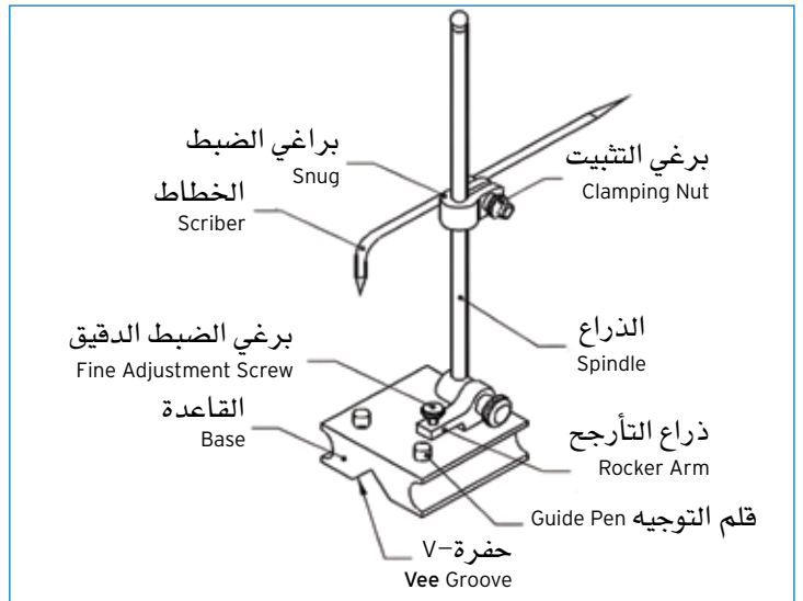
جهاز الشنكرة
