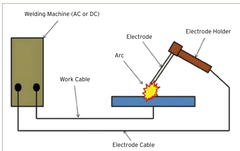
اللحام بالقوس المعدني
