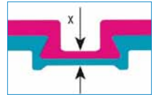
التجميع بالتشبيك
