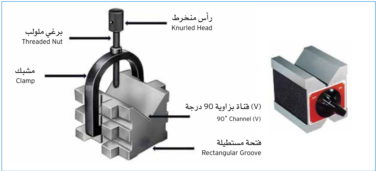
قوالب V
