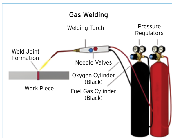
اللحام بالغاز (غاز الوقود)
