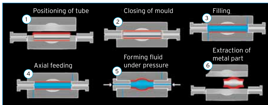
التشكيل الهيدروليكي
