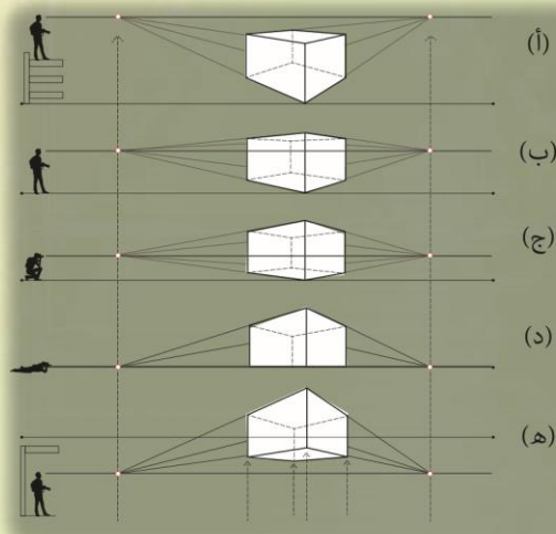
شكل (٣-أ، هـ) مستويات النظر المختلفة.
